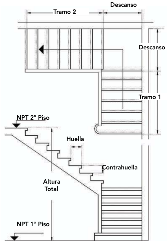
Figura 12 – 4: Planta y elevación tipo de una escalera de dos tramos en ángulo recto con descanso.
