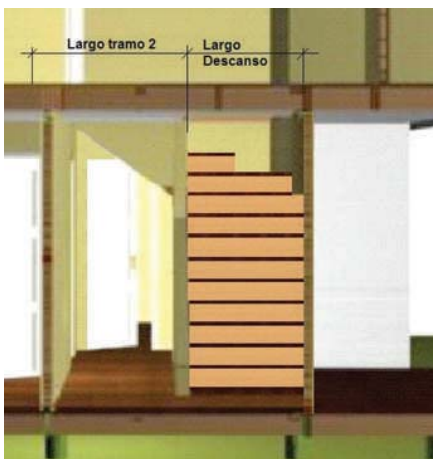
Figura 12 - 20b: Largo total de la escalera tramo 2.
