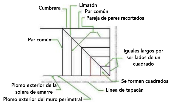
Figura 11-52: Vista en planta de las proyecciones de los elementos que conforman los cuadrados, destacándose los largos de los cuadrados que se forman.
