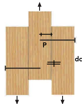
Figura 7- 16 : Resistencia lateral, cizalle simple.
