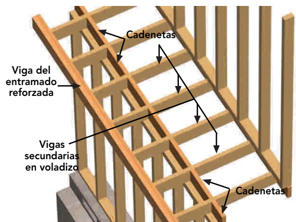
Figura 9 – 51: El entramado se encuentra en sentido perpendicular al voladizo. Envigado secundario de igual escuadría se ancla a la penúltima viga, la que se duplicare forzando dimensiones y largos según cálculo.
