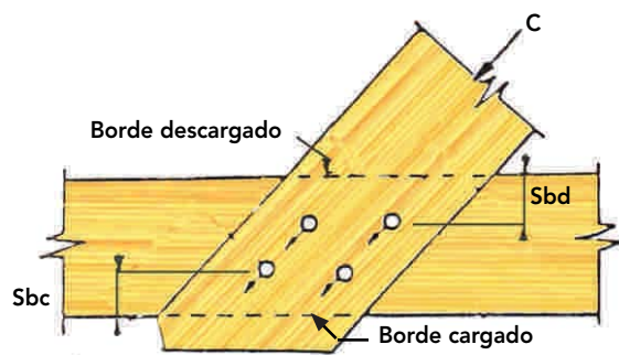
Figura 7 – 9 : Espaciamento mínimo entre un elemento de unión y el borde vecino.
