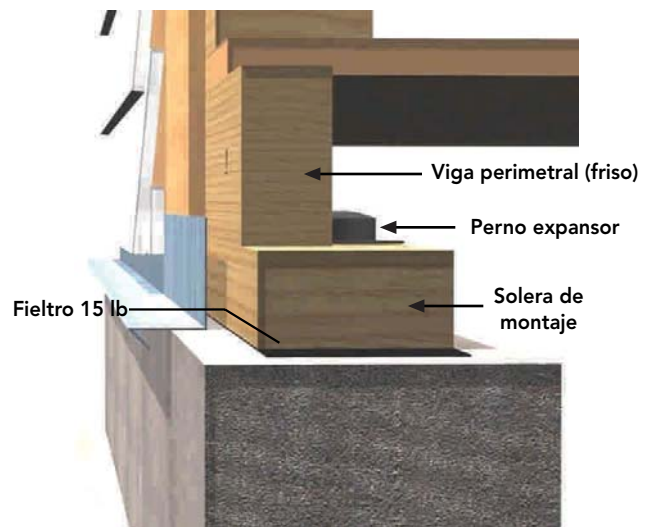
Figura 9 - 21: Solución de conexión de la viga perimetral al sobrecimiento, a través de una solera de montaje tratada con preservante CCA. Considera además, aislación entre ambos materiales con fieltro alquitranado. La solera está anclada al sobrecimiento mediante espárragos o pernos expansores cada 80 cm.
