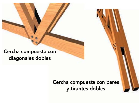
Figura 11-20: Las cerchas compuestas pueden tener los pares y tirantes dobles o pueden ser dobles, montante y diagonales.
