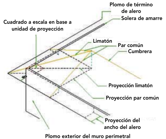
Figura 11-39: En rojo se destaca el cuadrado, proporcional a las proyecciones del limatón y par común anteriormente descrito, que será la unidad de proyección a utilizar. Nótese que se empieza a medir desde el borde exterior del tabique.
