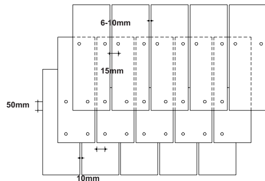
Figura 17-21A: Ubicación de fijaciones y distancia entre tejuelas.
