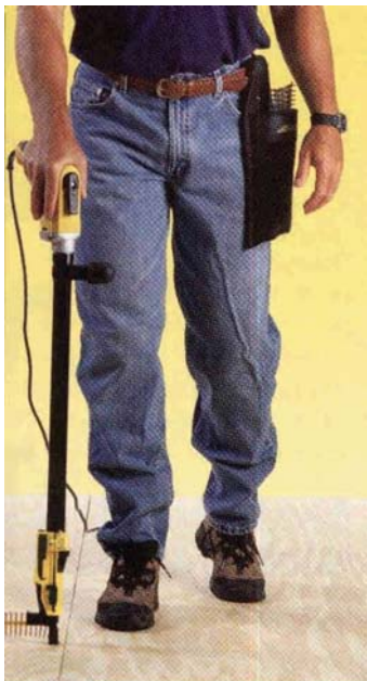
Figura 9 - 12: Taladro con extensión para atornillar tableros que arriostran la plataforma de un entramado de piso, a distanciamiento correspondiente.
