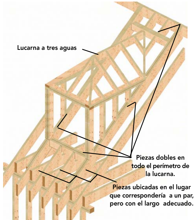
Figura 11- 75: Lucarna a tres aguas que interrumpe los elementos estructurales del diafragma inclinado y que requiere de refuerzos en el perímetro donde se recortaron las piezas de la estructura de techumbre.
