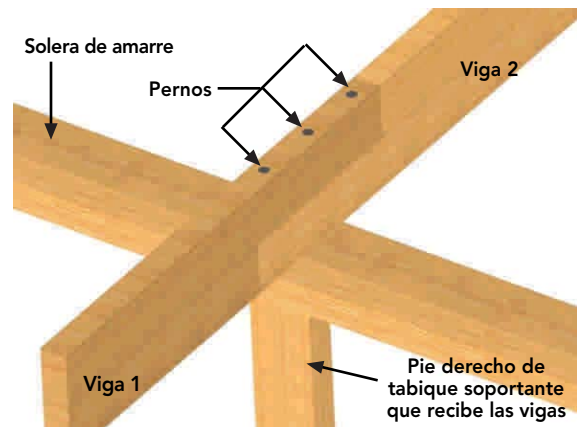
Figura 9 - 42: Empalme típico de dos vigas sobre un tabique estructural llamado ensamble en Entablatura , el cual consiste en ejecutar un corte tipo media madera y fijarlo con pernos, clavos, adhesivos o tarugos.
