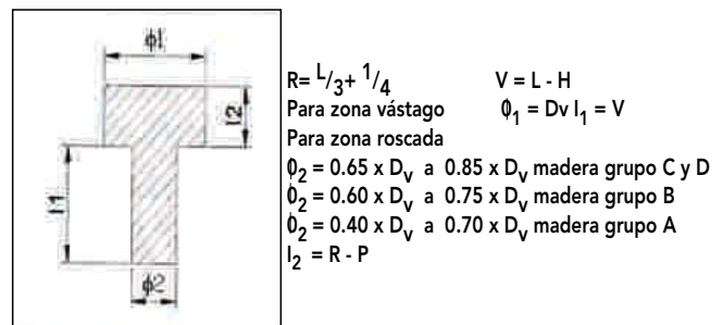
Figura 7-27: Perforación guía.
