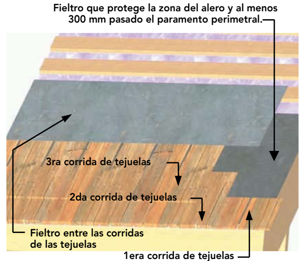
Figura 17-16: Disposición del fielto en la zona inicial y entre corridas de tejuelas.
