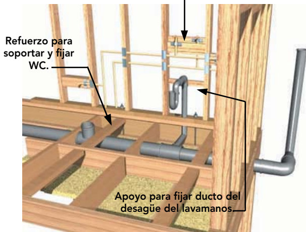
Figura 16-10: Ubicación de refuerzos a considerar en el diseño para fijar los ductos de las instalaciones.
