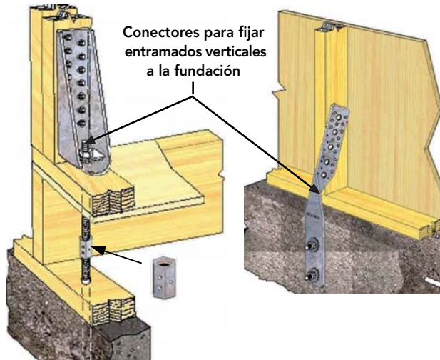
Figura 7- 32 : Alternativas de conectores metálicos para fijar elementos verticales como tabiques o pie derecho.
