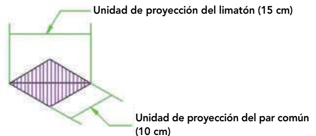
Figura 11-40: Detalle de la unidad de proyección (cuadrado), del cual se deducen la unidad de proyección del limatón y par común respectivamente.
