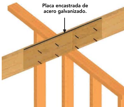
Figura 9 - 40: Empalme a tope sobre tabique soportante, reforzado con placa encastrada de acero galvanizado (distancia entre fijaciones según cálculo).
