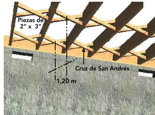
Figura 9 - 7: Vista desde abajo de la plataforma de madera anclada sobre una fundación continua. Crucetas con distancia máxima a 1,2 m según proyecto.
