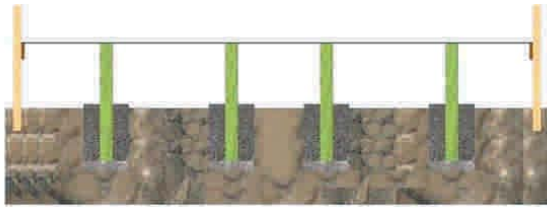
Figura 8 - 47: Hormigonado de los cimientos y nivelación de la cabeza de los pilotes.
