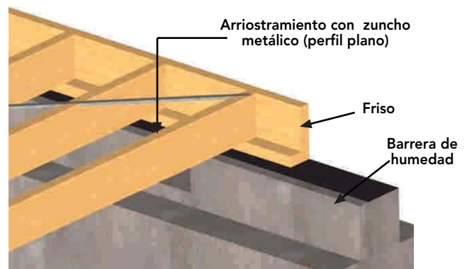
Figura 9 - 10 : Zuncho metálico, pletina de ancho 20 mm y espesor 2,5 mm para plataforma de primer piso, anclada a la fundación continua.
