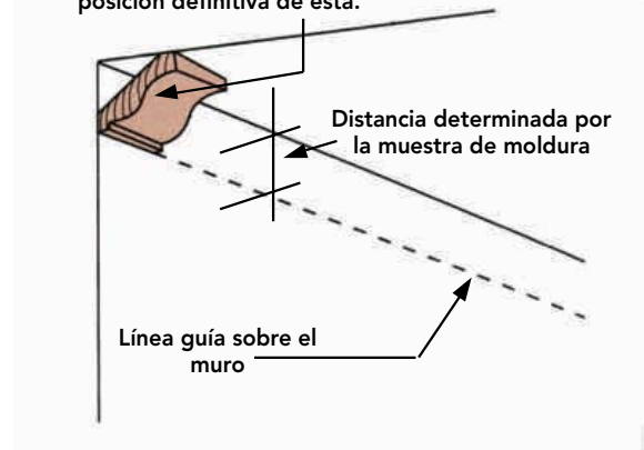
Figura 21-12 : Trazado de la línea guía para la correcta instalación de la moldura.
