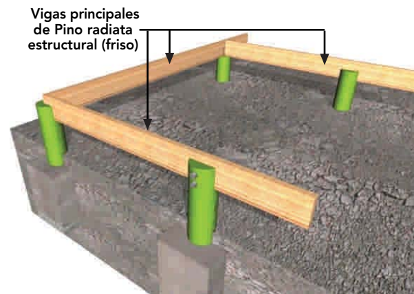
Figura 9 - 30: En el ejemplo, se muestra el friso que remata el contorno del entramado de piso en una solución de fundación aislada.
