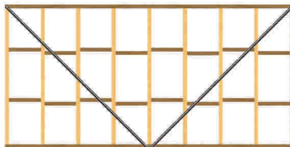
Figura 10-22a: Tabique soportante arriostrado por medio de tensores en barras de acero plano.
