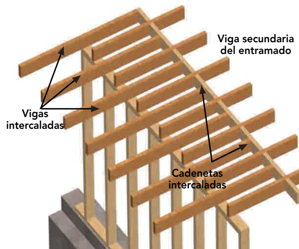
Figura 9 – 50: El voladizo se encuentra en el sentido del entramado de las vigas. En este caso, se intercalaron nuevas vigas entre las existentes, anclándolas a la viga cabezal, dimensiones y largos según cálculo.
