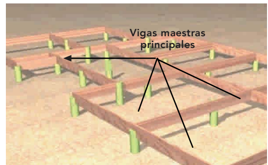
Figura 8 - 51: Fundación aislada, materializada considerando los aspectos y criterios de cálculo.
