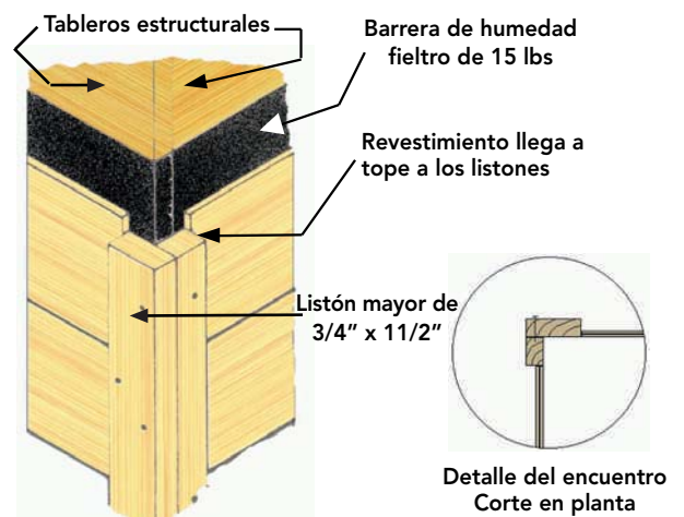
Figura 18 - 18: El clavado de los listones es en forma de zig-zag como se observa en la figura, correspondiendo uno como fijación a la estructura y el siguiente como fijación al listón de encuentro.
