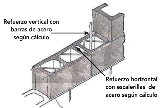
Figura 8 - 34 : De mucha importancia resulta proteger los bloques de hormigón en sus paramentos exteriores de la humedad por capilaridad, adquirida por contacto con el terreno o por lluvia directa.
