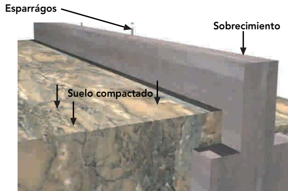
Figura 8 - 52: Rigurosa compactación del suelo, donde se apoya la plataforma de hormigón.
