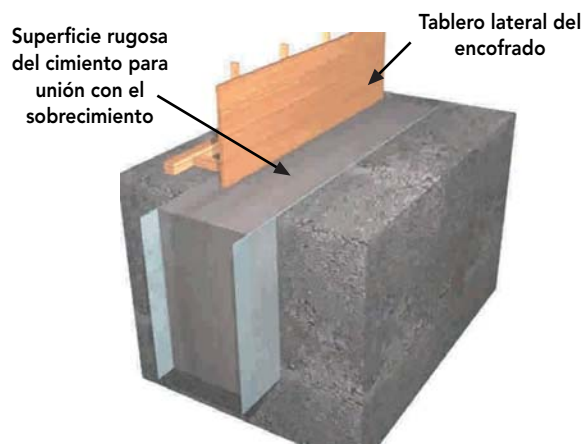
Figura 8-29: Instalación inicial del encofrado para la materialización del sobrecimiento.
