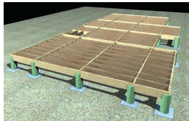
Figura 9 – 4: Vigas de Pino radiata estructural, de escuadrías según cálculo, normalmente de 2" x 8" o 2" x 10" que conforman el entramado de piso en fundación aislada sobre pilotes de madera.
