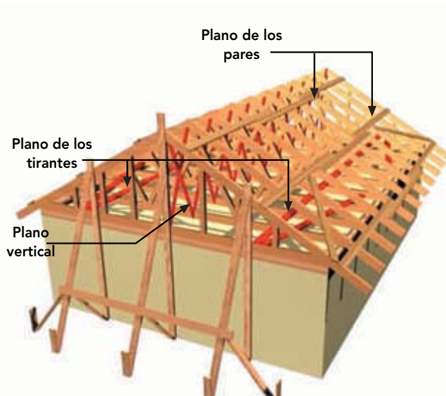
Figura 11-30: Planos en los que se deben realizar los arriostamientos de las cerchas.
