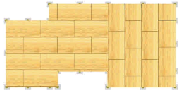
Figura 9 - 13: El plano de planta de construcción debe especificar la disposición de los tableros estructurales: contrachapado fenólico (terciado estructural) o de hebras orientadas (OSB).
