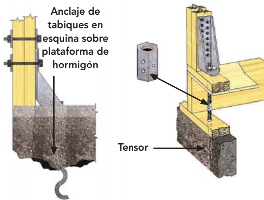
Figura 10 – 40: Anclaje que permite privilegiar el traspaso directo de los componentes sísmicos, desde el pie derecho a la fundación y no a la solera inferior, como usualmente se soluciona (anclaje aplicado normalmente en tabiques soportantes de esquina).
