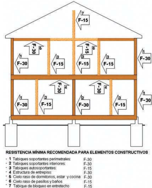
Figura 15 – 25: Requerimiento mínimo de resistencia al fuego por tipo de elemento de construcción y servicio, para viviendas unifamiliares no pareadas ni adosadas.
