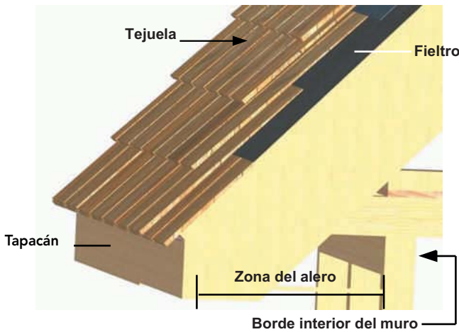
Figura 17-15: Fielto debe cubrir al inicio de la techumbre el alero y al menos 300 mm pasados el borde interior del muro perimetral.
