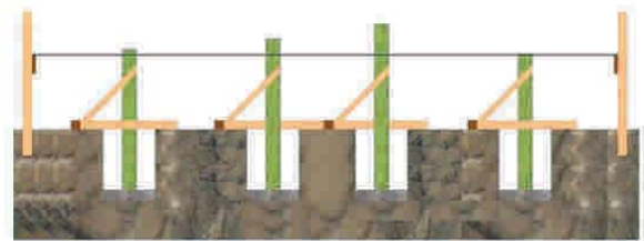
Figura 8 - 46: Control geométrico de los pilotes, planimetría y altimetría según plano. Arriostramiento de pilotes para cuidar la verticalidad durante el hormigonado del cimiento.
