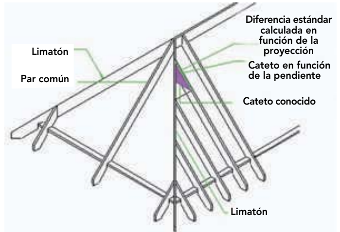
Figura 11-54: Deducción del cálculo de la diferencia estándar, en base a la distancia entre pares y la pendiente de la techumbre.
