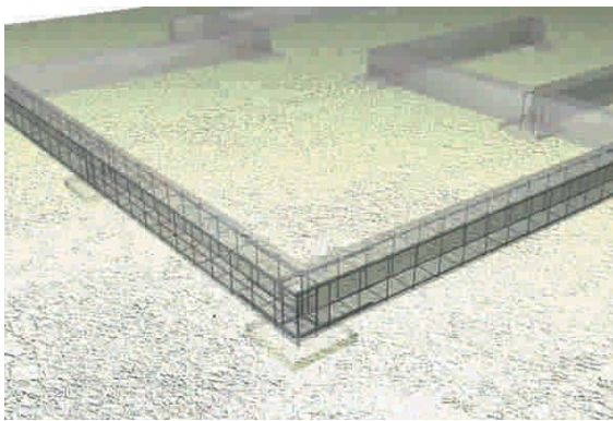
Figura 8 - 13: Viga de fundación que amarra los pilotes de hormigón y recibe el muro perimetral de la vivienda.
