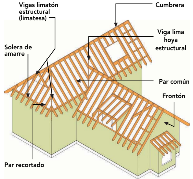
Figura 11-37: Vista en perspectiva que muestra la ubicación de los elementos definidos.
