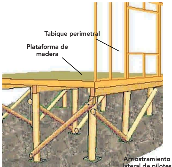
Figura 8 - 49 : Arriostamiento de pilotes según cálculo estructural.
