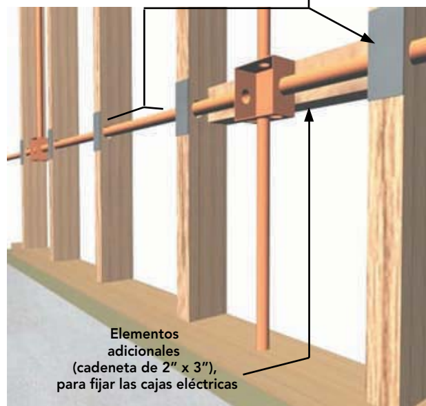
Figura 16 - 5: Consideraciones para la instalación, fijación y protección de ductos y accesorios.
