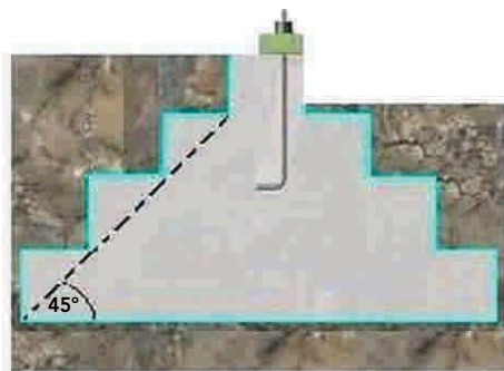
Figura 8 - 18 : Caso de fundación en terrenos aluviales.
