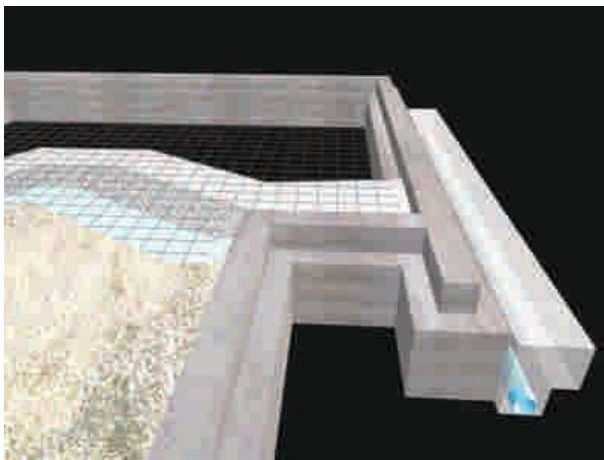
Figura 3 - 5: Tubo de P.V.C perforado adyacente al cimiento y que colecta las aguas, evacuándolas al punto más bajo.
