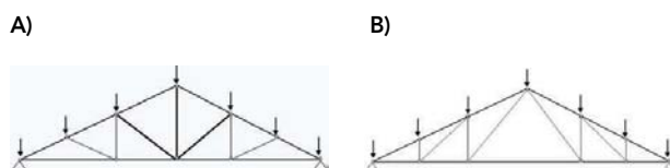
Figura 11- 24: Esquema de cerchas que muestran en función del sentido de las diagonales, si estarán solicitadas a compresión (A) o tracción (B).
