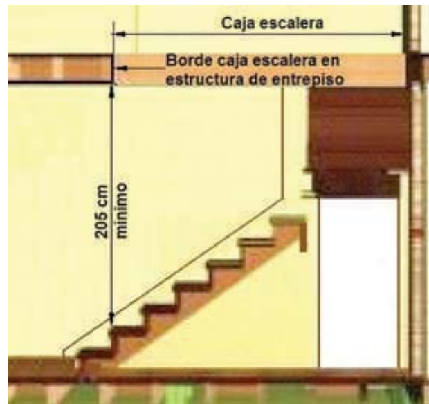
Figura 12 - 21: Altura libre vertical mínima entre huella y cielo raso. También puede considerarse todo elemento superior sobre la cabeza de quien sube o baja por la escalera.
