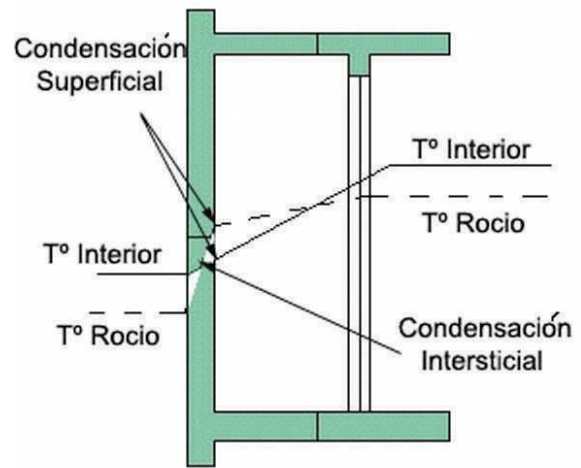
Figura 13 – 17: Condensación superficial e intersticial en clóset.
