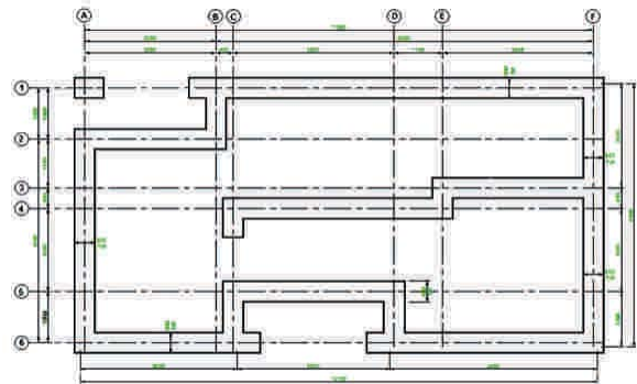
Figura 8 - 24: Plano de excavaciones de la vivienda prototipo.
