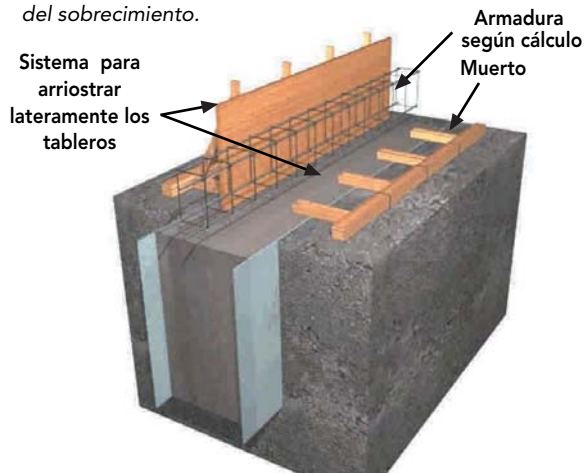
Figura 8 - 30: Instalación de la armadura para el sobrecimiento, en caso que el cálculo así lo indique.
