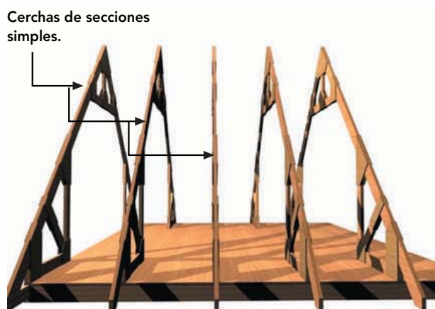
Figura 11-19: Vista en elevación de cerchas simples.
