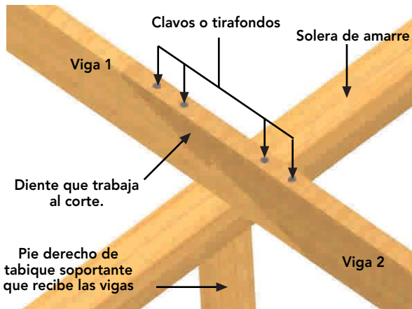
Figura 9 – 43: Empalme de dos vigas llamado Rayo de Júpiter sobre tabique estructural, en el cual las vigas se cruzan como en la solución Entabladura , pero incorporando un diente que trabajará al corte. Se puede utilizar en su fijación pernos o clavos.
