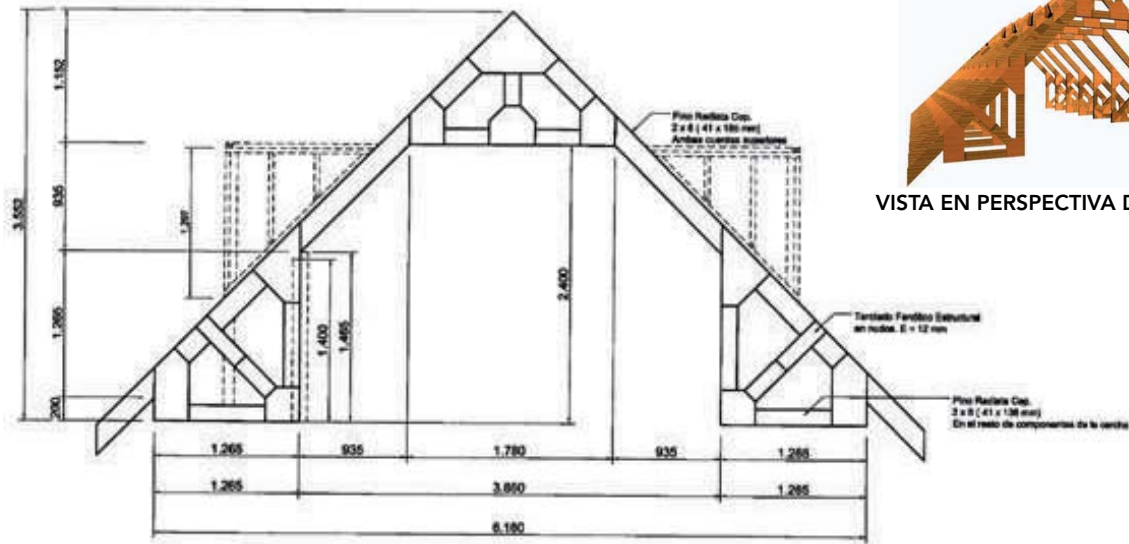
PLANO DE DETALLE DE CERCHA TIPO (a)
