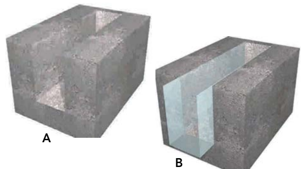
Figura 8 - 25: En la figura A la excavación ha sido controlada geoméricamente y en la B se ha dispuesto polietileno de e = 0,5 \text{ mm} en las paredes de la excavación.
