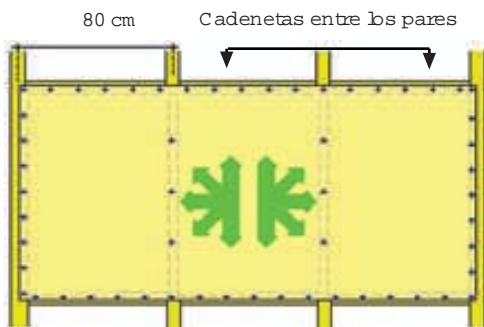
Figura 11-64 : Clavado de placa a los pares, de cerchas o diafragma inclinado, ubicados cada 80 cm y a cadenas ubicadas en el perímetro de la placa.
