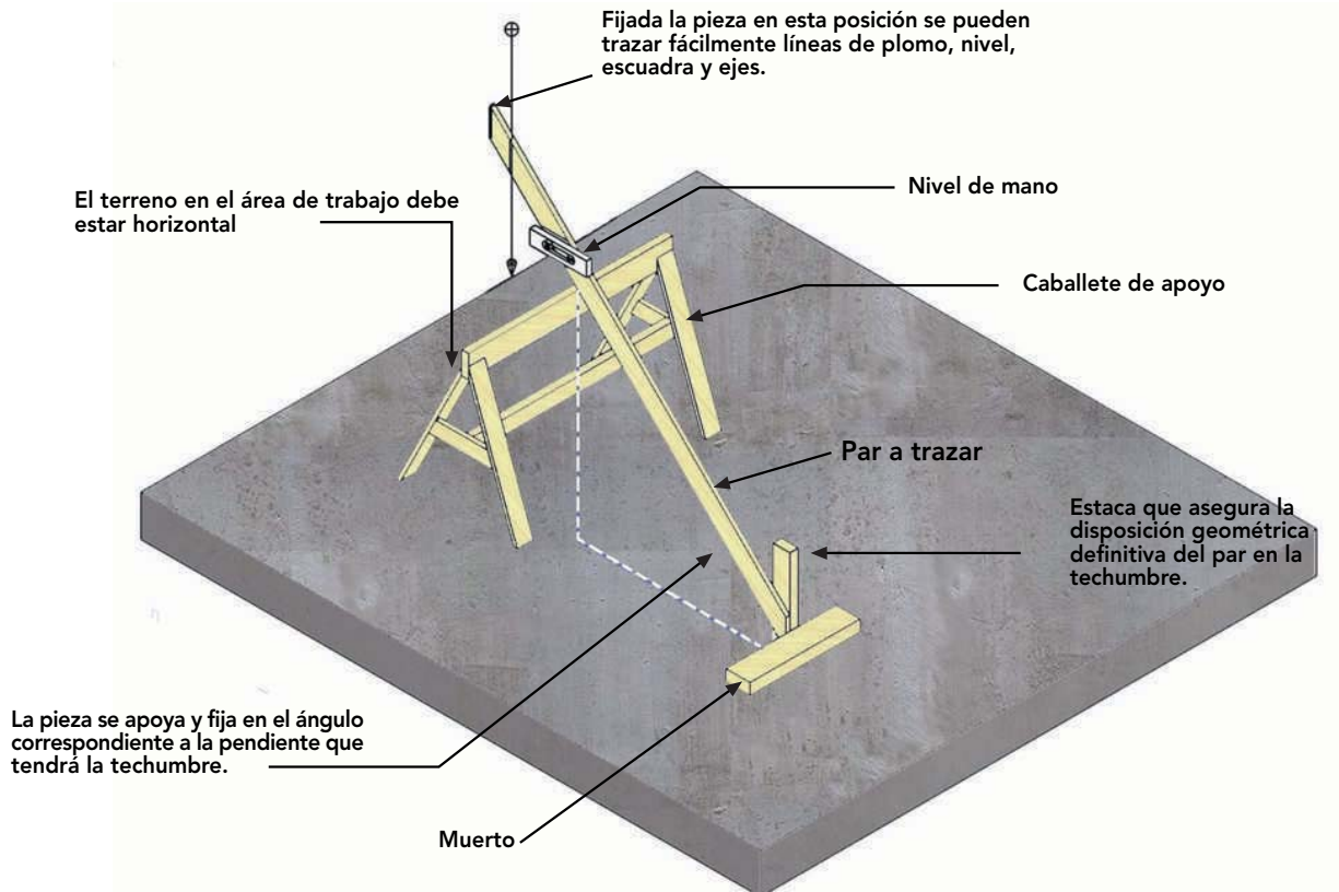
Figura 11 -57: Ejemplo de un lugar de trabajo con las condiciones mínimas para obtener cortes adecuados en los elementos. Se debe simular la pendiente que tendrá el elemento en el techumbre, modificando la altura del caballete y la distancia a que debe ir el muerto para realizar los cortes de manera exacta.
